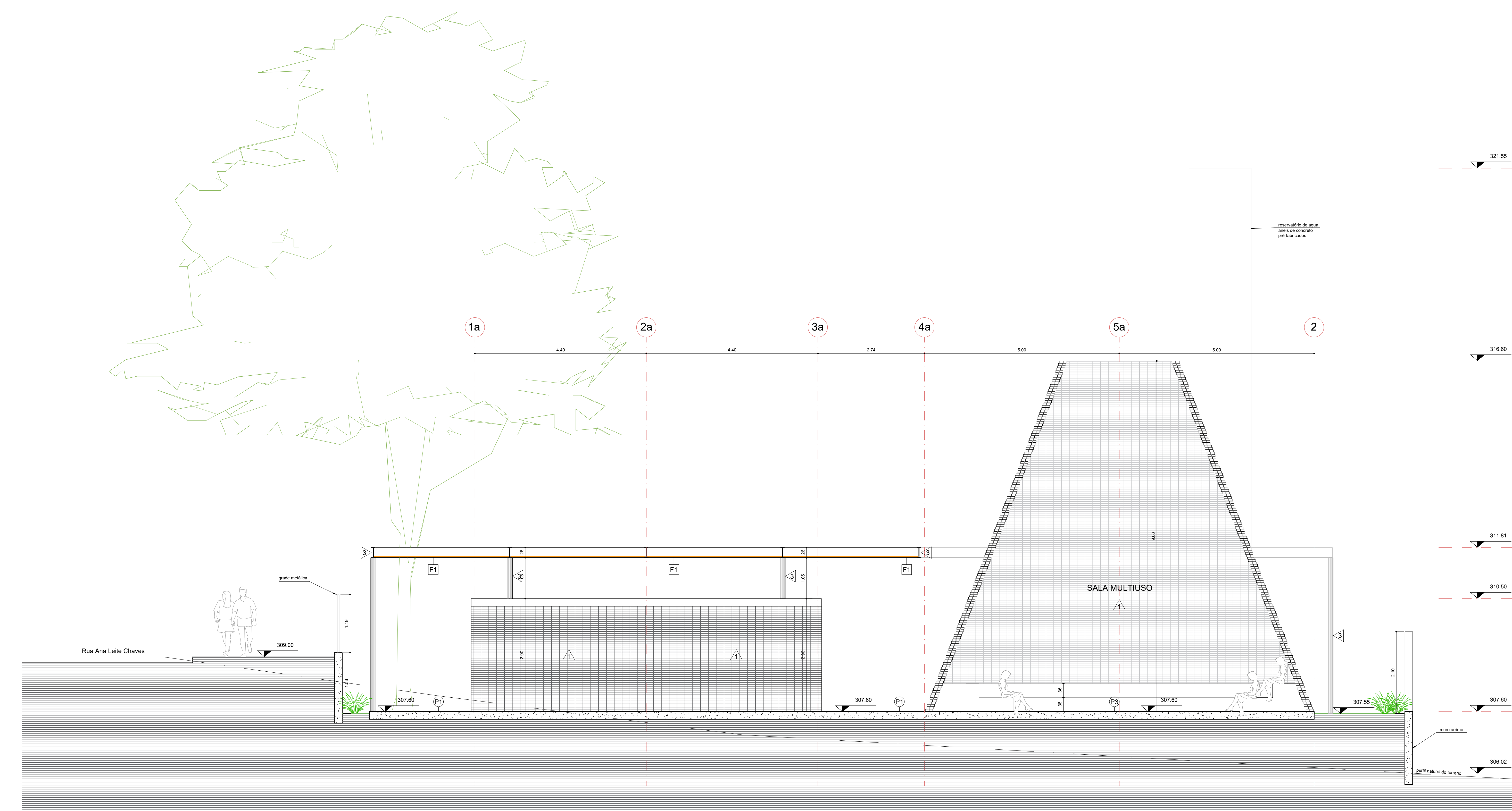
CORTE DD
