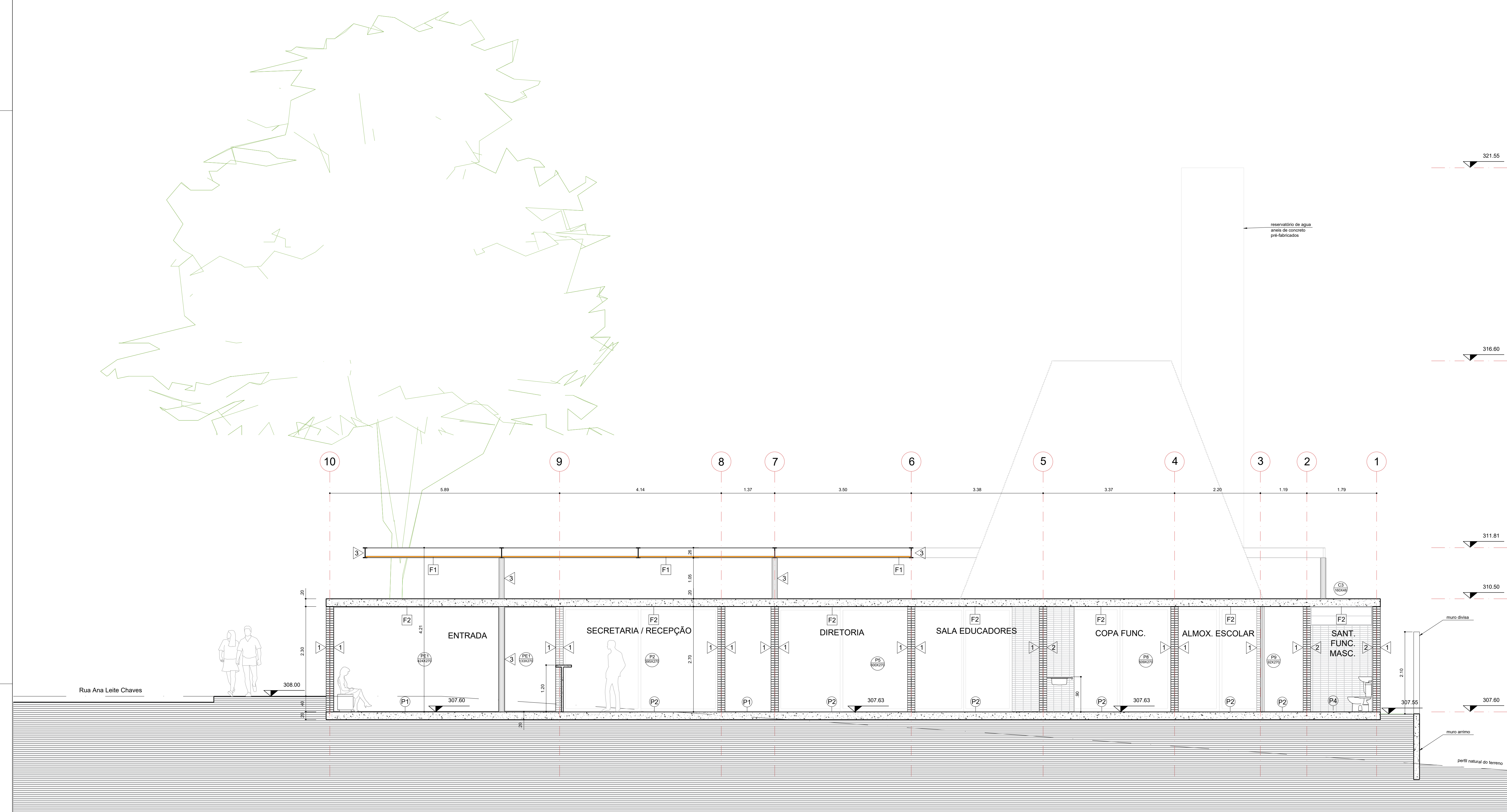
CORTE CC
