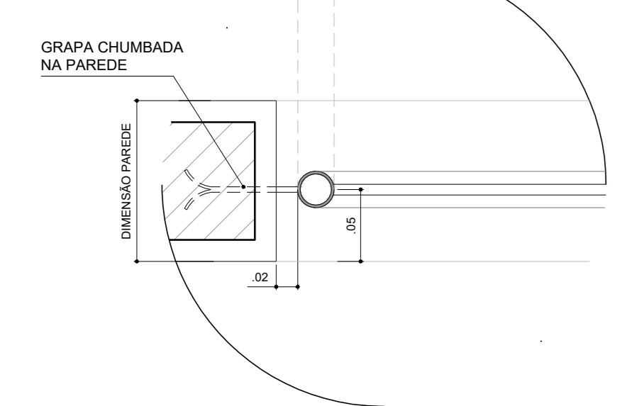
DETALHE 07 ESCALA 1/5
